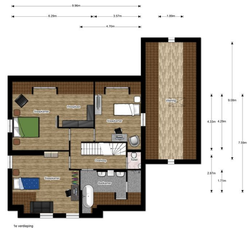
1e verdieping
